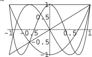
Slika 1.2 Čebiševljevi polinomi
