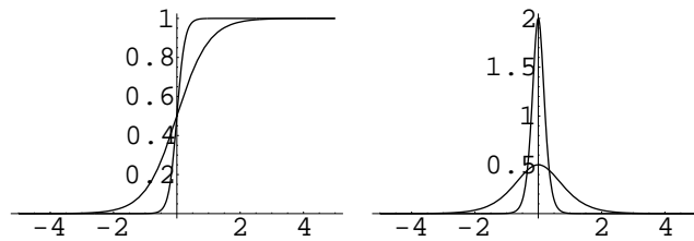
Slika 2.2 Funkcije S_\epsilon(t) i S'_\epsilon(t)
