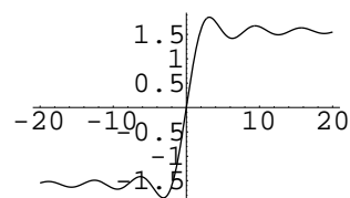
Slika 2.1 Sinus integralni
