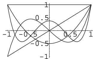
Slika 1.1 Legendreovi polinomi
